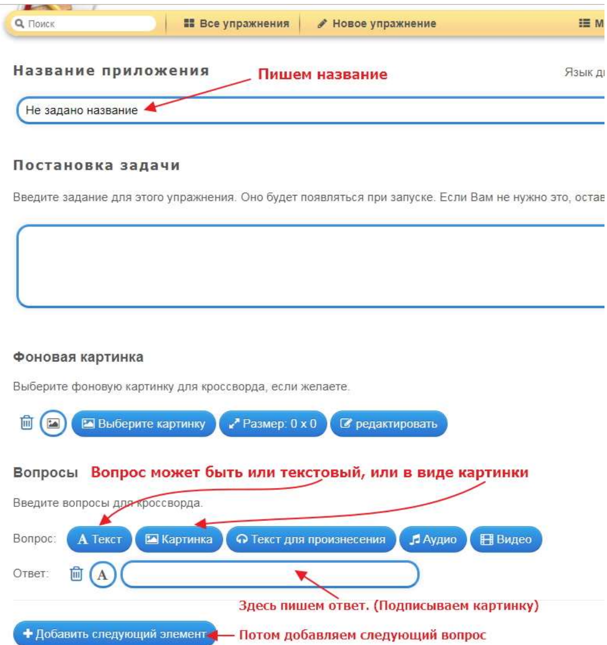
Рис.1 Создание кроссворда
